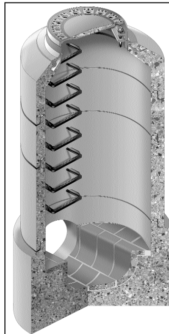
econorm® - ein ausgereiftes und sicheres Schachtsystem. ✎
